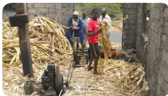
Ilustração 70: Trapiches tradicional (à esquerda) e motorizado. Fonte: Internet e Autor.
